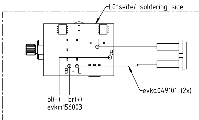
Blotschaltbild/ block diagram
