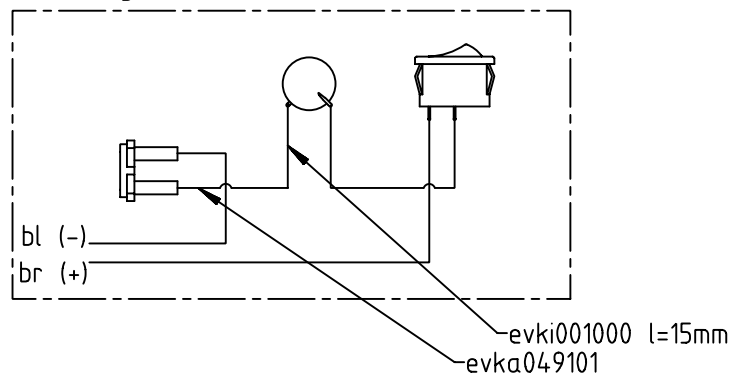
Blockschaltbild / block diagram
