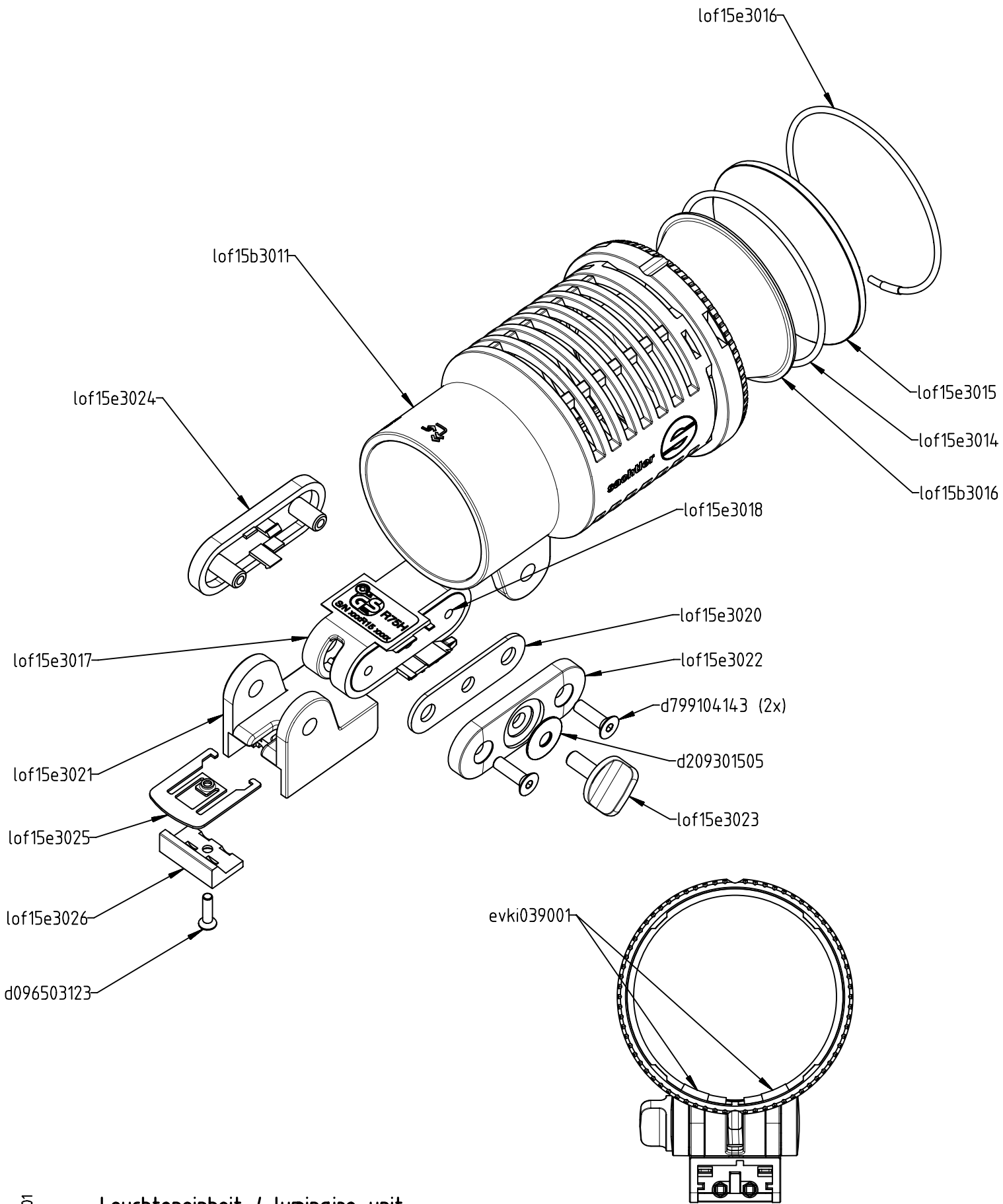
Leuchteneinheit / luminaire unit für / for R75H
