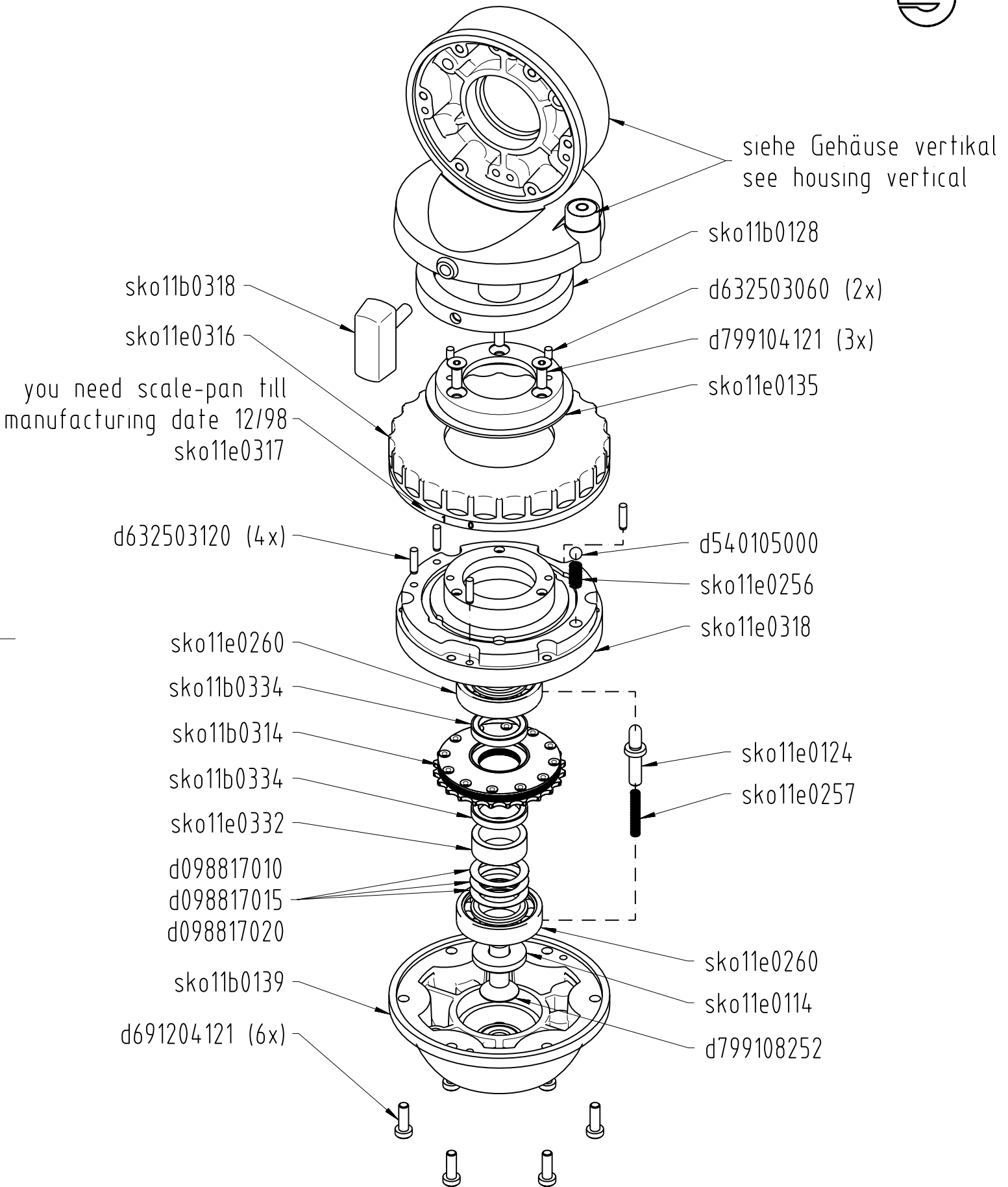
Halbkugel mit Dämpfungspaketen Ball assembly with fluid modules
